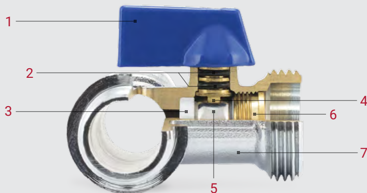
КРАН ТРЁХХОДОВОЙ ДЛЯ СМА PF BWV 361
