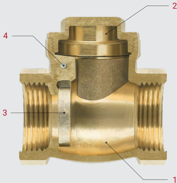
КЛАПАН ОБРАТНЫЙ ДИСКОВЫЙ ГОРИЗОНТАЛЬНЫЙ PF CV 249
