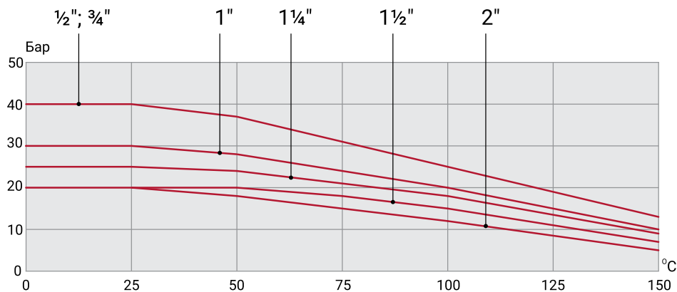
ГРАФИК ЗАВИСИМОСТИ МАКСИМАЛЬНОГО РАБОЧЕГО ДАВЛЕНИЯ ОТ ТЕМПЕРАТУРЫ
