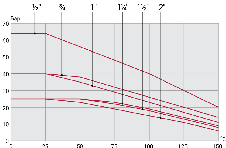
ГРАФИК ЗАВИСИМОСТИ МАКСИМАЛЬНОГО РАБОЧЕГО ДАВЛЕНИЯ ОТ ТЕМПЕРАТУРЫ
