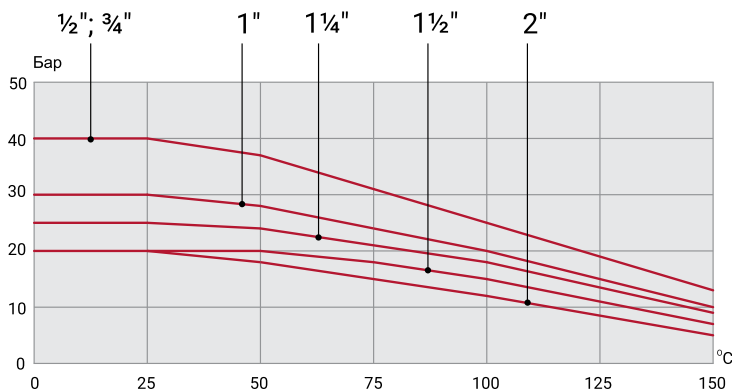
ГРАФИК ЗАВИСИМОСТИ МАКСИМАЛЬНОГО РАБОЧЕГО ДАВЛЕНИЯ ОТ ТЕМПЕРАТУРЫ
