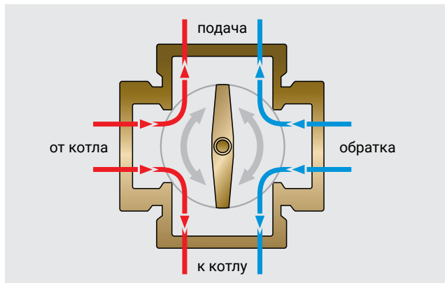
ПРИНЦИП РАБОТЫ 4-Х ХОДОВОГО КЛАПАНА:
