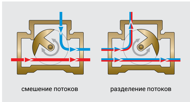
ПРИНЦИП РАБОТЫ 3-Х ХОДОВОГО КЛАПАНА:
