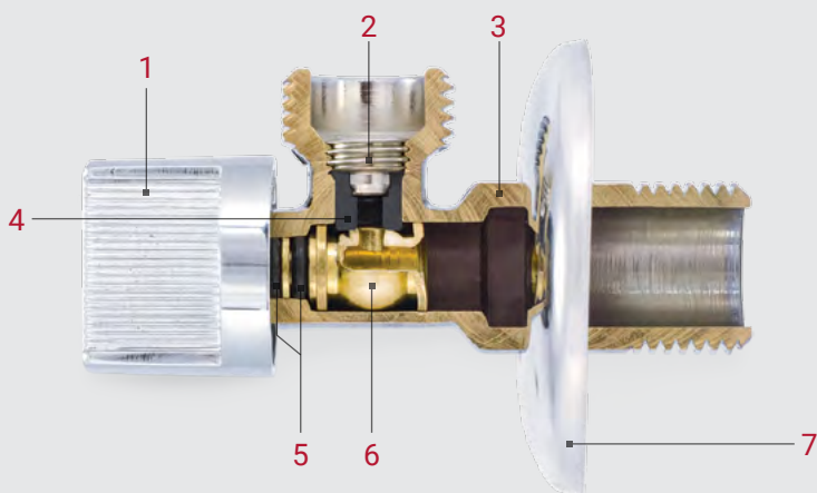
КРАН УГЛОВОЙ ХРОМИРОВАННЫЙ PF BAV 357
